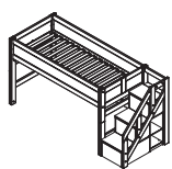
HALBHOHES BETT MIT TREPPE H 128 x B 257 x T 102 Lichte Höhe 89 CM
