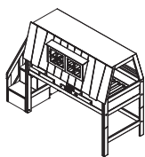
HALBHOHES BETT HANGOUT MIT TREPPE H 195 x B 261 x T 107 Lichte Höhe 89 CM
