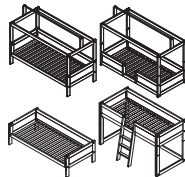
4-IN-1 BETT FÜR STOFFDACH H 128/161 x B 207 x T 102/124 Lichte Höhe 2 / 25 / 89 CM
