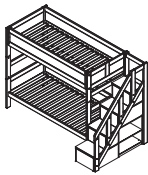
ETAGENBETT FAMILY MIT TREPPE H 177 x B 257 x T 102/132 Lichte Höhe 25 CM Anstand zwischen den Betten 104 CM
