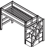
MITTEL-HOCHBETT MIT TREPPE H 152 x B 257 x T 102 Lichte Höhe 113 CM
