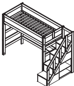
HOCHBETT MIT TREPPE H 177 x B 257 x T 102/132 Lichte Höhe 139 CM
