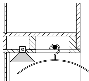
Nischenüberbau: Detail der Mantelstange und Beleuchtung. Niche bridge: Detail of hanging rail and lighting.
